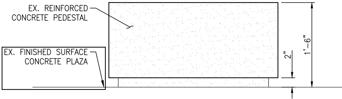
ELEVATION
